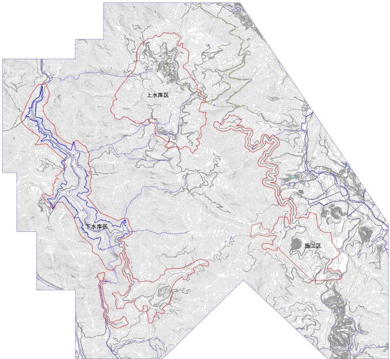
福建永安抽水蓄能电站站址保护范围图
